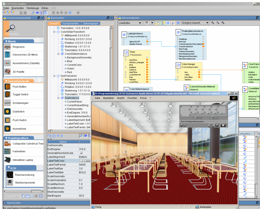
Abbildung 5: 3D-Autorenwerkzeug CONTIGRABUILDER und erzeugte VRML97-Beispielanwendung
